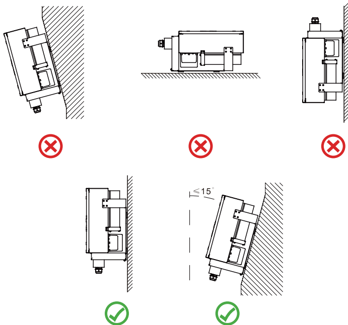
图4.2 安装角度
