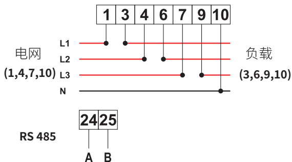
图7.5 正泰电表
