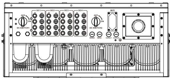
图1.2 底视图
