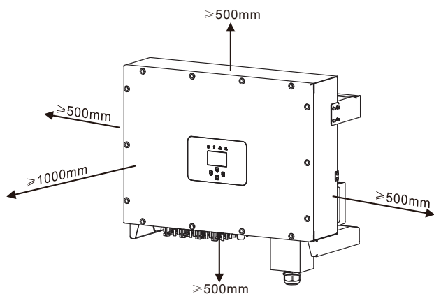
图4.3 安装间隙
