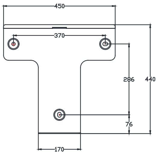
图 4.4 支架尺寸
